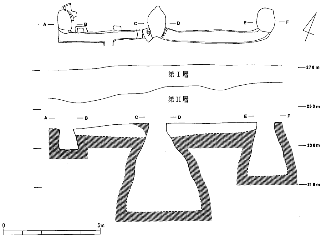
1. ピット15、16、19平面図および断面図
